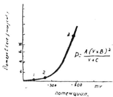
Зависимость склонности сплава к коррозии от его потенциала.
