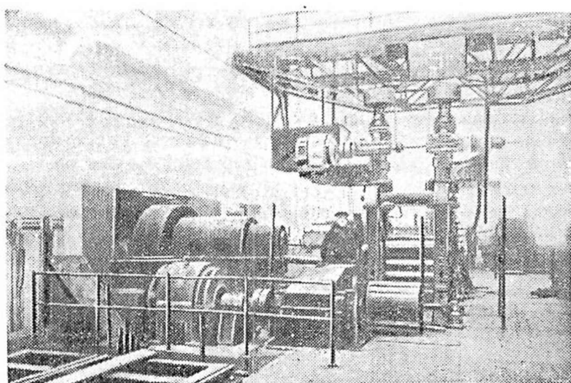
Недавно в Институте закончено строительство лабораторного корпуса. В настоящее время заканчивается монтаж новой лаборатории прокатки. НА СНИМКЕ: комбинированный прокатный стан, установленный в новой лаборатории.
