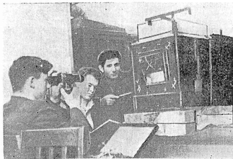
На снимке: студенты в лаборатории металлургических печей определяют оптическим пирометром температуру в печи. Фото Л. СТОЧЕКА.
