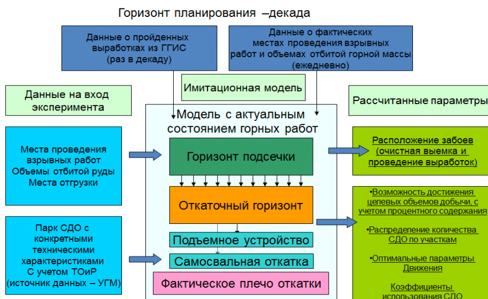
Рисунок 2 – Концептуальная схема системы имитационного моделирования, при горизонте планирования декада
