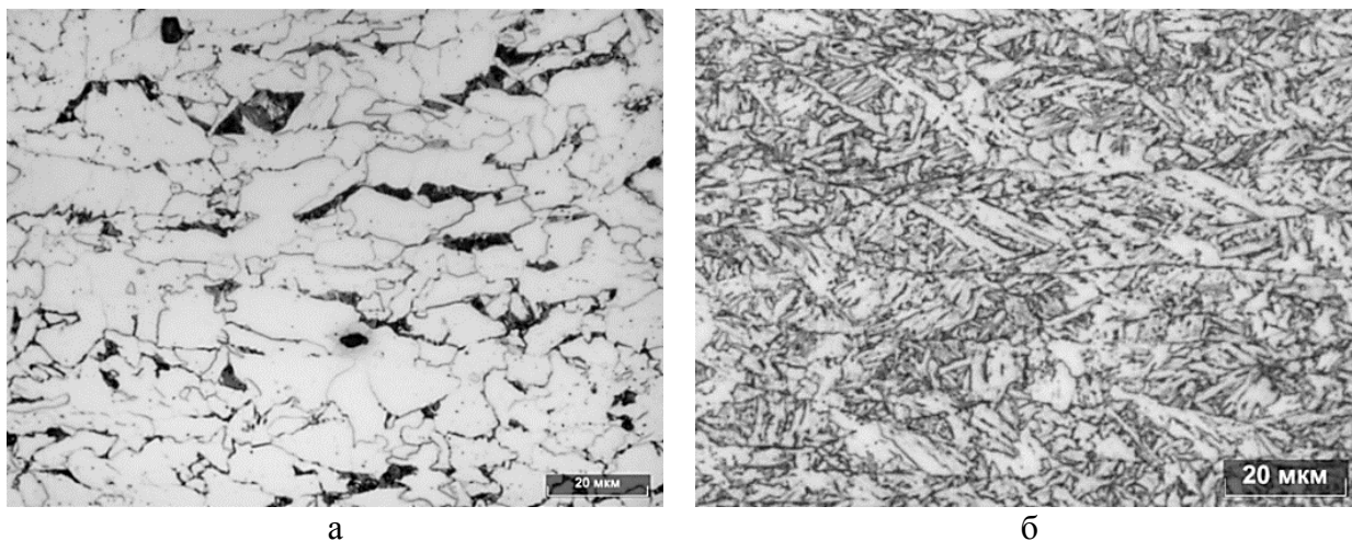
а) С390П (В)-1; б) С390П (В)-2
