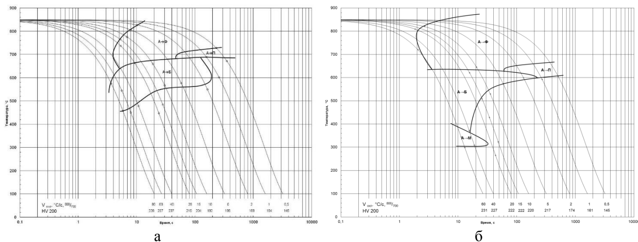
Рисунок 7 – Термокинетические диаграммы распада аустенита
