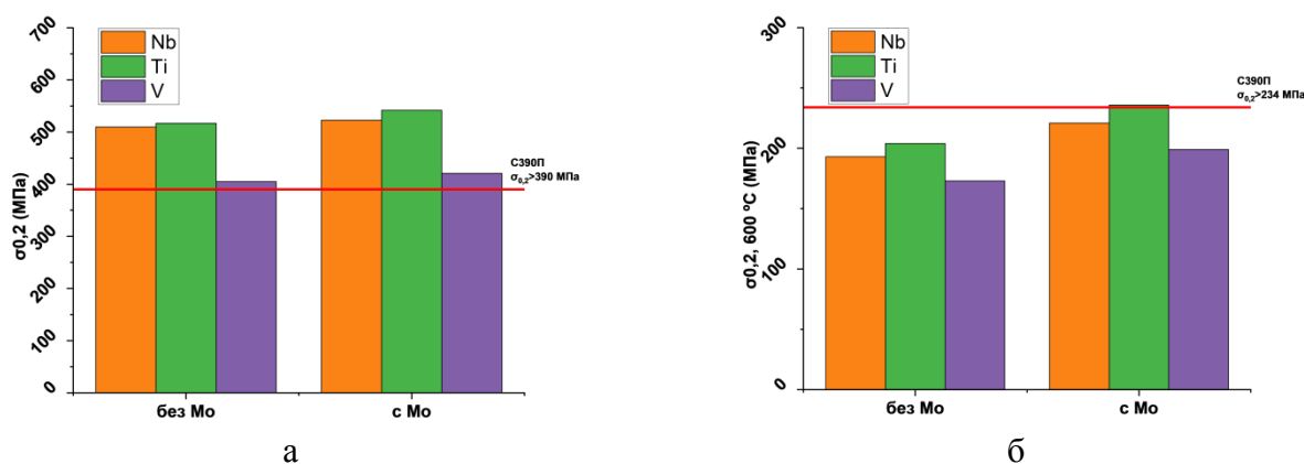
Рисунок 3 – Влияние химического состава на изменение предела текучести
