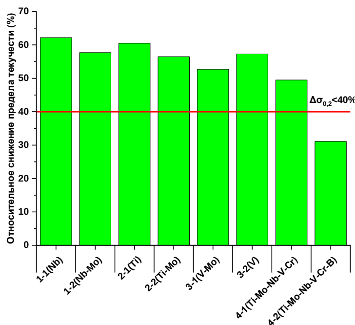
Рисунок 4 – Относительное разупрочнение лабораторных плавков первой серии выплавки
