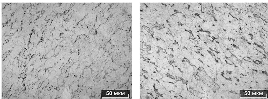
а) 5 (Cr-Nb-V-B); б) 6 (Cr-Nb-V); в) 7-1 (Cr-↑Nb-V), после КП+УО (550)+О(550); г) 7-2 (Cr-↑Nb-V), после КП+УО (500)+О(500)
