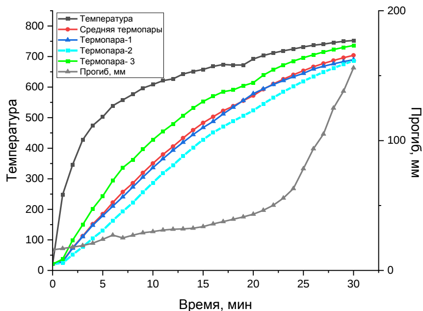
Рисунок 12 – Графики изменения температуры в огневой камере печи и величины соответствующего прогиба для опытного образца сварной балки, изготовленного из рулонного проката С390П
