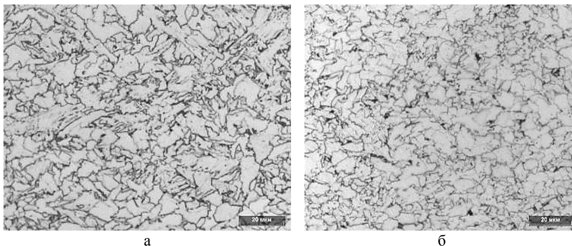
а) С390П10; б) С390П-12
