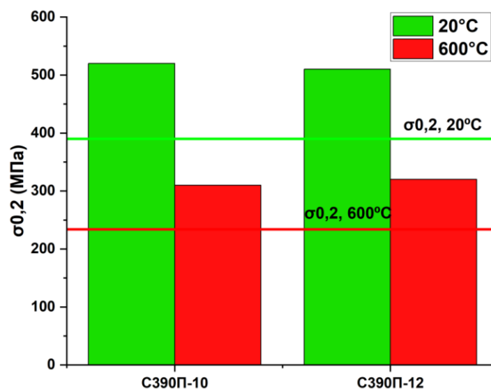
Рисунок 10 – Предел текучести промышленного рулонного проката С390П при комнатной и повышенной температуре (600 °С)
