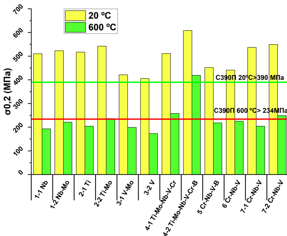
Рисунок 6 – Предел текучести проката, произведенного в рамках лабораторных экспериментов, при испытании при комнатной температуре и 600 °C
