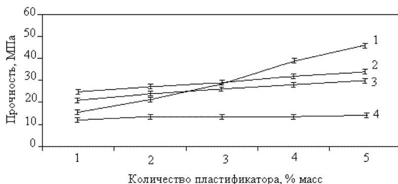
Рисунок 3 - Зависимость прочности (на сжатие) прессовок из смеси сплава ВК8 от количества и вида пластификатора: 1- ПВА, 2 – ПЭГ, 3 – ПЭГ-ПВА, 4 – СК.
