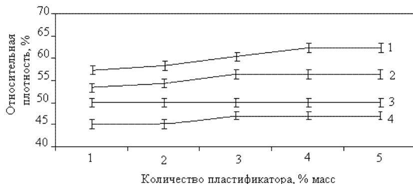
Рисунок 1 - Зависимость плотности прессовок из сплава ВК8 от количества и вида пластификатора: 1- СК, 2 – ПВА, 3 – ПЭГ-ПВА, 4 – ПЭГ.
