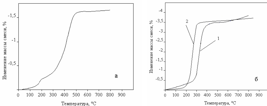
Рисунок 7. Термогравиметрические кривые разложения в атмосфере водорода в составе твердосплавной смеси ВК8: а – СК, б – ПЭГ (1) и ПВА (2).
