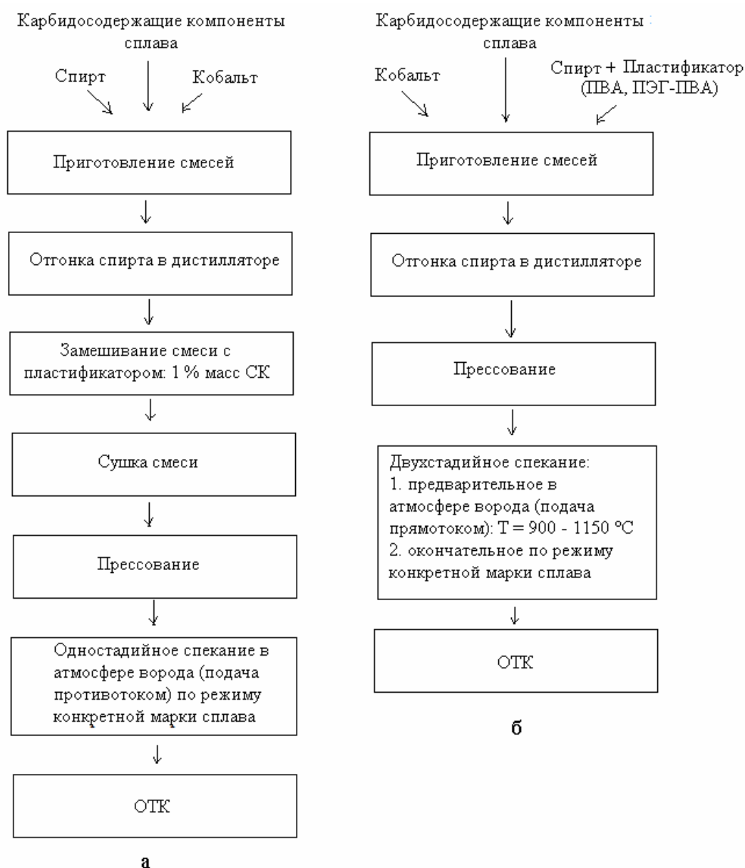
Рисунок 9. Схемы производства твердосплавной продукции: а – действующая в промышленности; б – предложенная.
