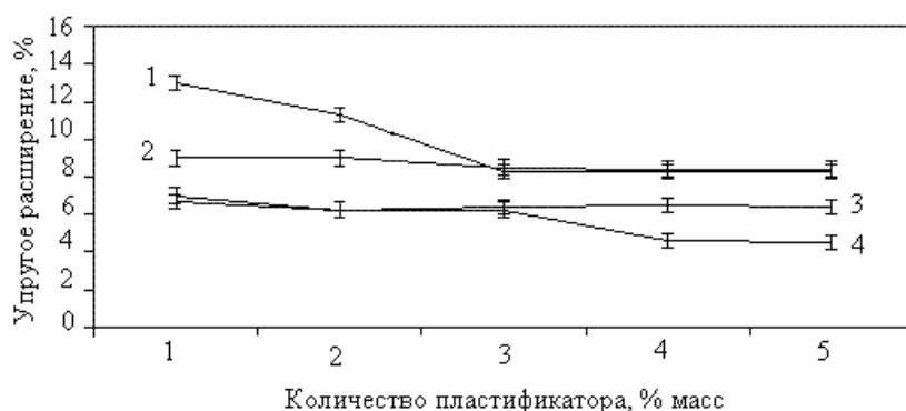
Рисунок 2 - Зависимость упругого расширения прессовок из сплава ВК8 от количества и вида пластификатора: 1- ПЭГ, 2 – ПЭГ-ПВА, 3 – ПВА, 4 – СК
