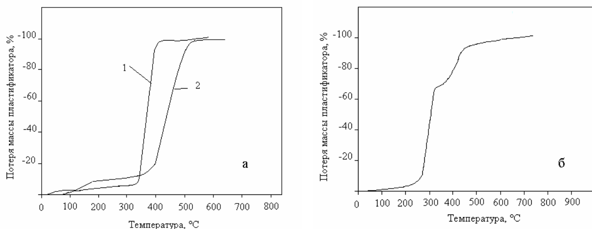
Рисунок 6. Термогравиметрические кривые разложения в атмосфере водорода: а – ПЭГ (1), СК (2); б - ПВА.
