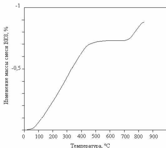
Рисунок 8. Термогравиметрическая кривая разложения твердосплавной смеси ВК8 в атмосфере водорода.
