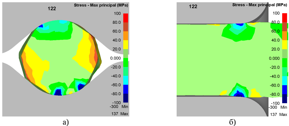
Рисунок 5.11 – Максимальные главные напряжения при ковке в вырезных радиусных бойках
