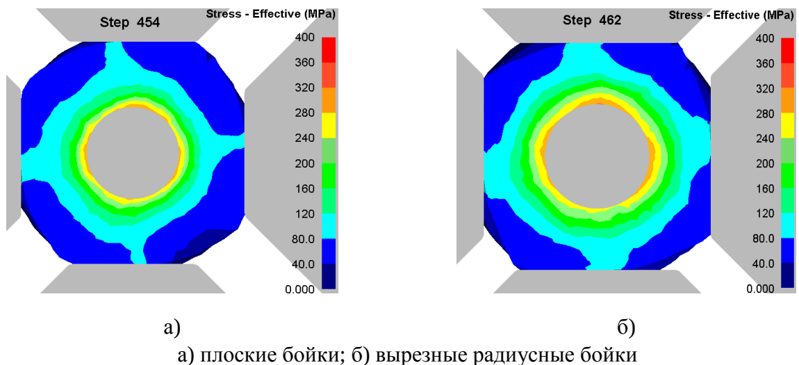
Рисунок 5.37 – Распределение интенсивности напряжений (разрез по заходному участку)
