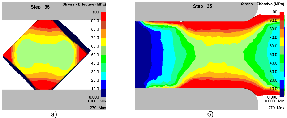
Рисунок 5.10 – Интенсивность напряжений в конце процесса
