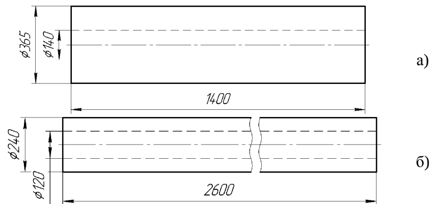
а) размеры заготовка; б) размеры итоговой поковки
