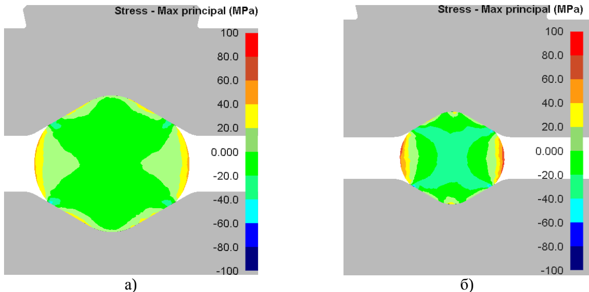
а) бойки для начальной стадии процесса б) бойки для финальной стадии процесса Рисунок 5.22 – Распределение главных напряжений при использовании вырезных бойков
