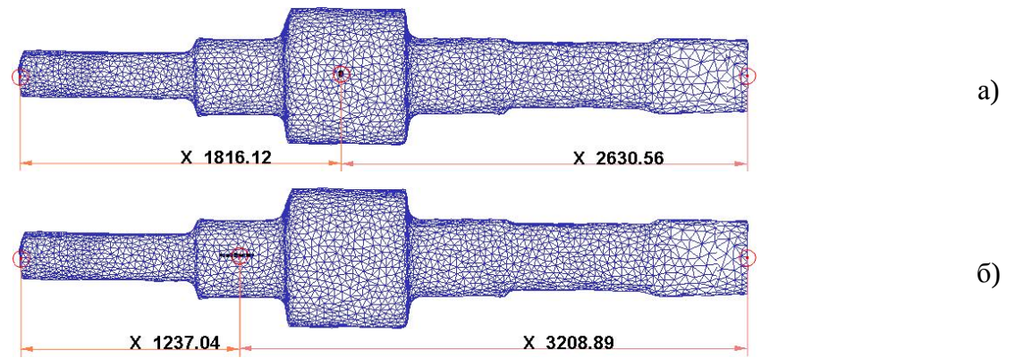
а) центральная часть заготовки, б) передняя часть заготовки
