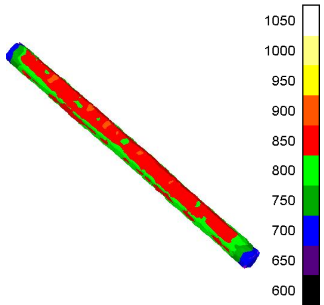
Рисунок 5.26 – Получение профиля восьмигранного поперечного сечения
