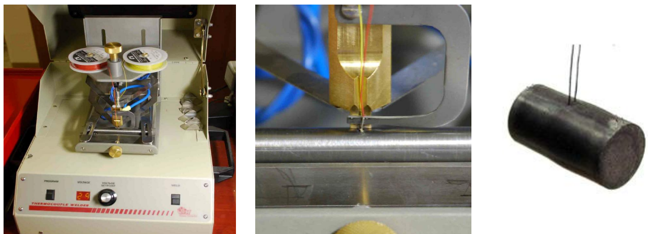
Рисунок 2.19 – Процесс крепления термопар
