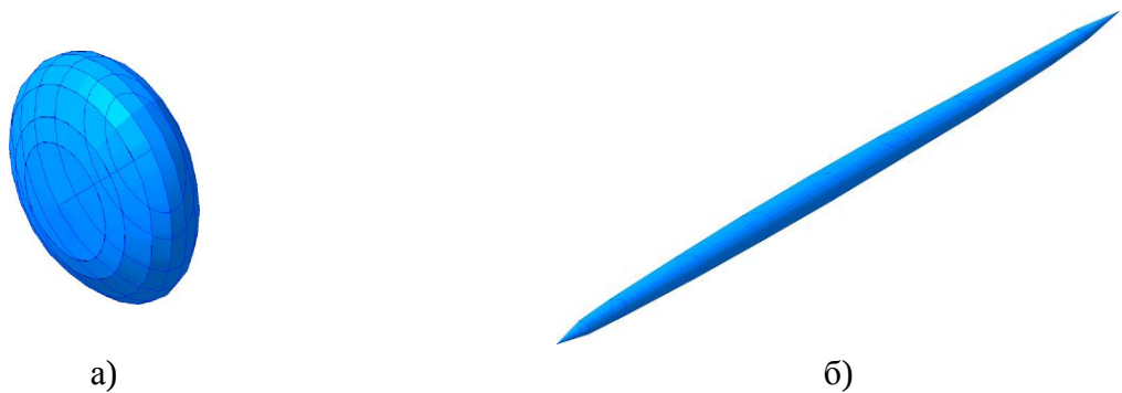
а) центральная часть заготовки, б) передняя часть заготовки Рисунок 3.61 – Формоизменение сфер после итоговой протяжки
