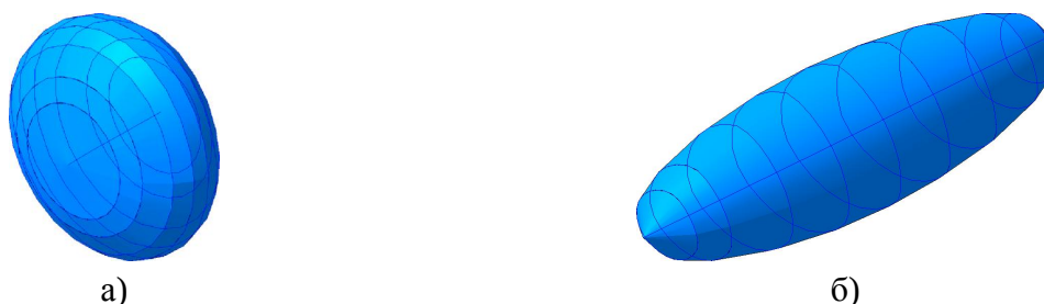
Рисунок 3.40 – Формоизменение сфер после протяжки до диаметра 775 мм
