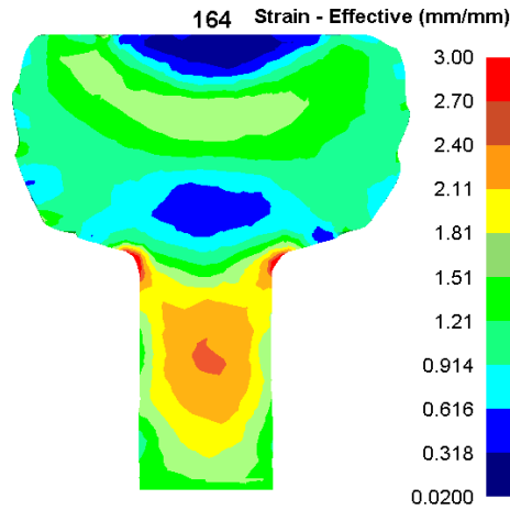
Рисунок 3.15 – Распределение накопленных деформаций по поверхности билета после осадки
