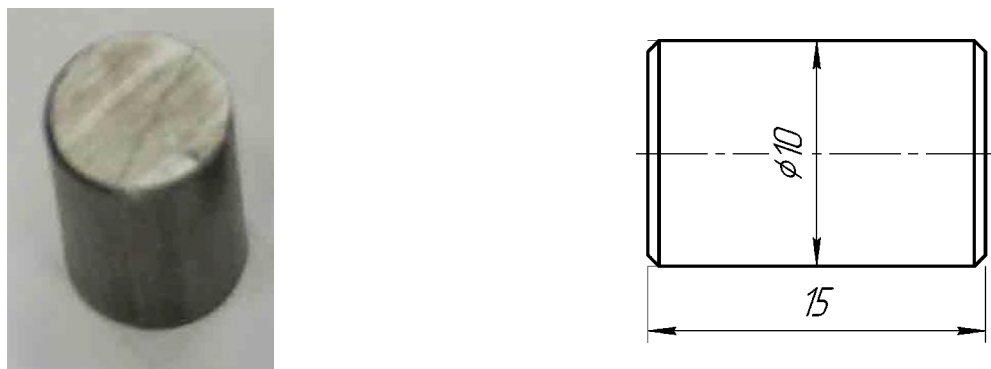
Рисунок 2.18 – Внешний вид и размеры применяемых образцов
