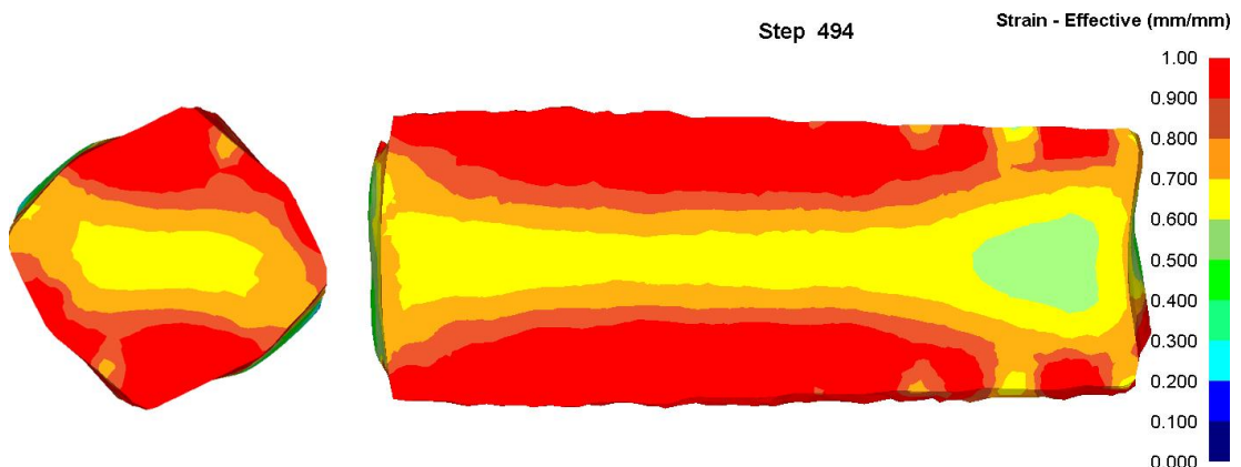
Рисунок 2.35 – Распределение накопленных деформаций при использовании бойков со скрещивающимися рабочими поверхностями после второго прохода
