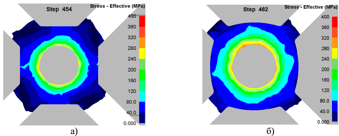
а) плоские бойки; б) вырезные радиусные бойки
